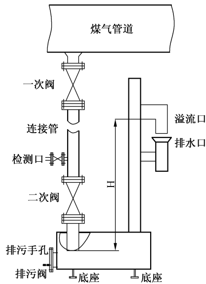
图 A.3 卧式水封式煤气排水器结构示意图
